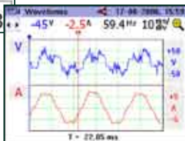
Visualice las formas de onda para la verificación y configuración del equipo.
